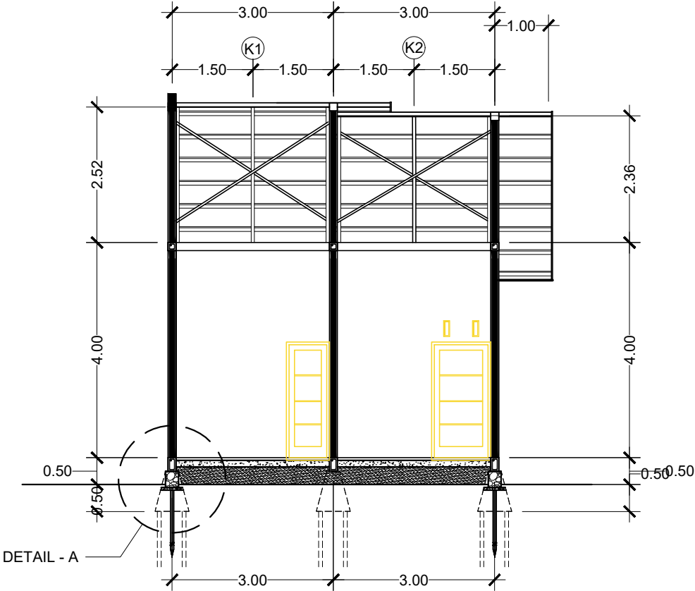
POTONGAN_A SKALA 1 : 100
