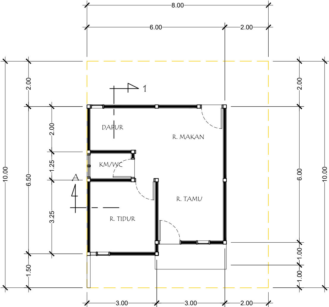
DENAH TYPE 36 SKALA 1 : 100
