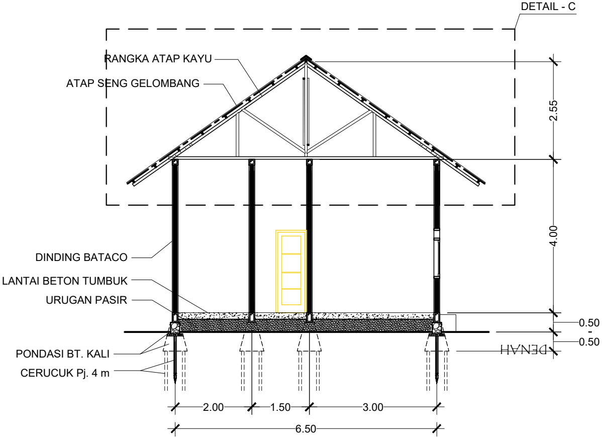
POTONGAN_1 SKALA 1 : 100
